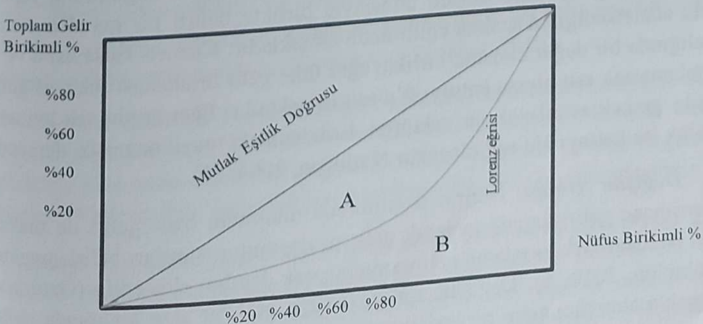
Grafik 1. Lorenz Eğrisi
